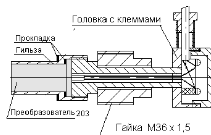
Рисунок 13 – комплект монтажных частей для ПП-200-203
